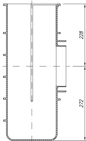
SECCION A-A
