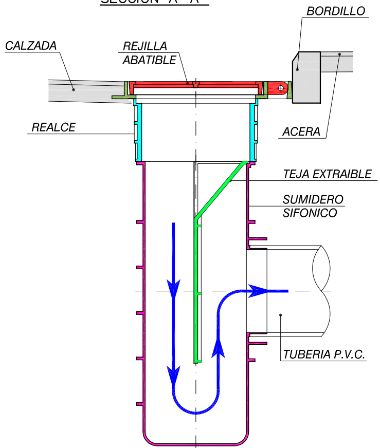
DETALLE SUMIDERO-REALCE-REJILLA
