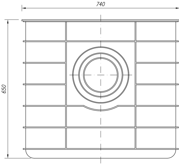
ALZADO VISTA POR "A"
